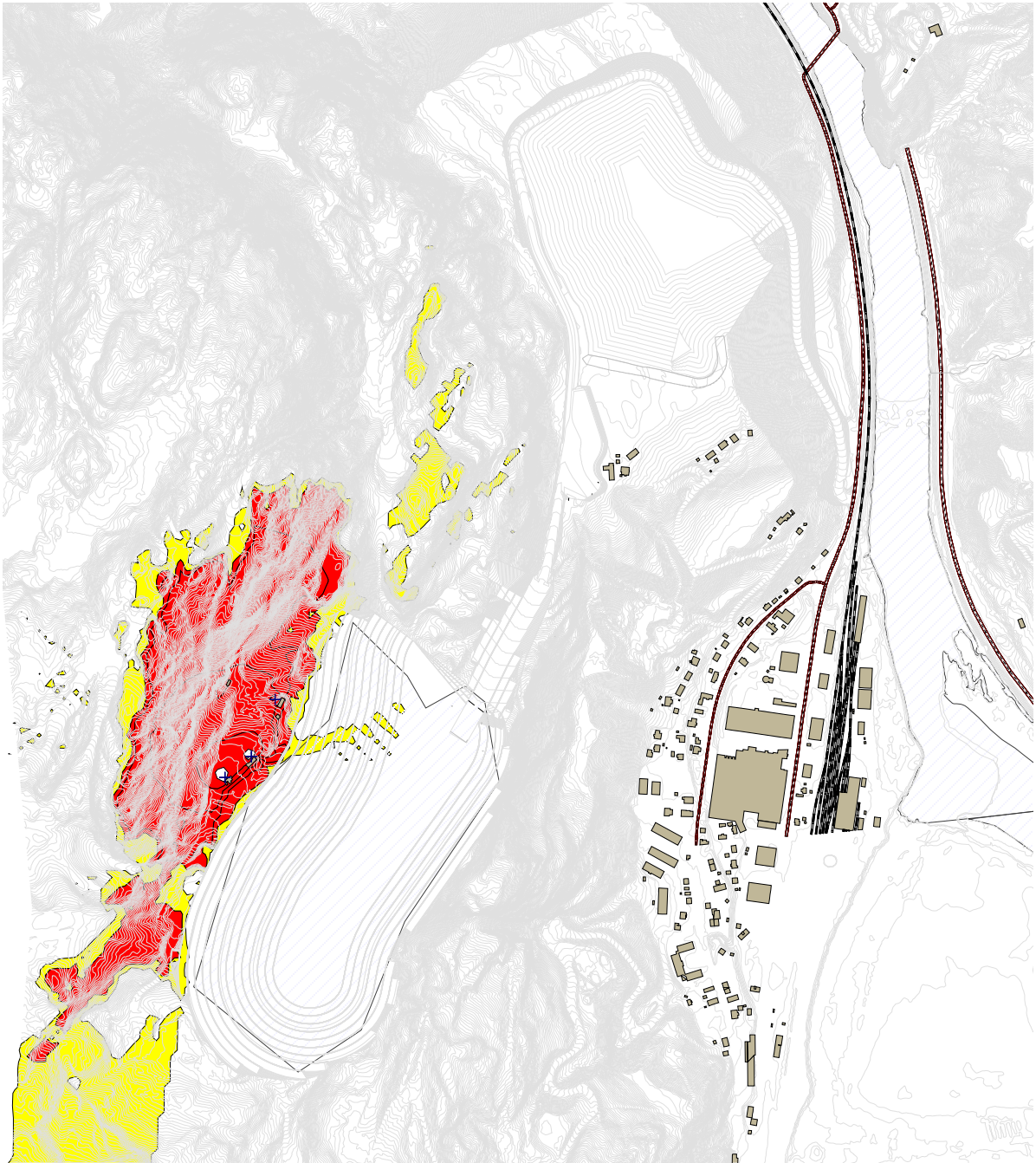
Figur 3: Støysonekart skytebane i 4 meters høyde. Gul sone L_{A_{fmax}} 65 dB - 75 dB, Rød sone L_{A_{fmax}} \geq 75 dB
