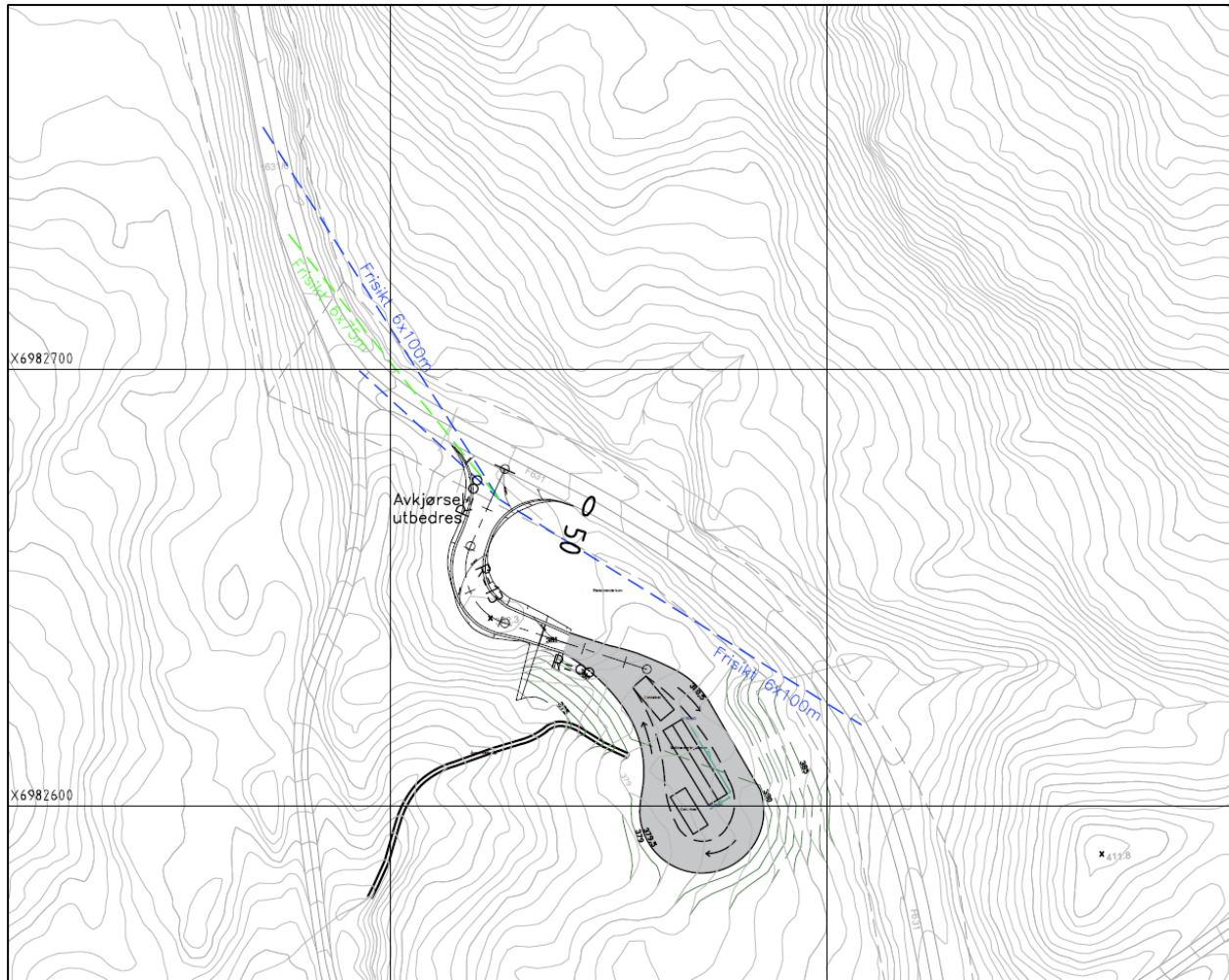
Figur 18: Utvidelse av avkjørsel
