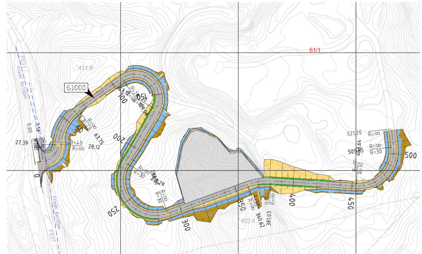
Figur 19: Planlagt ny veg til deponiet.
