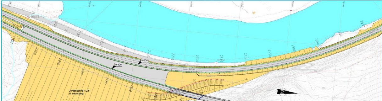
Figur 9 Utbedring av eksisterende E6 med vegfylling ut i Gaula og behov for erosjonssikring.
